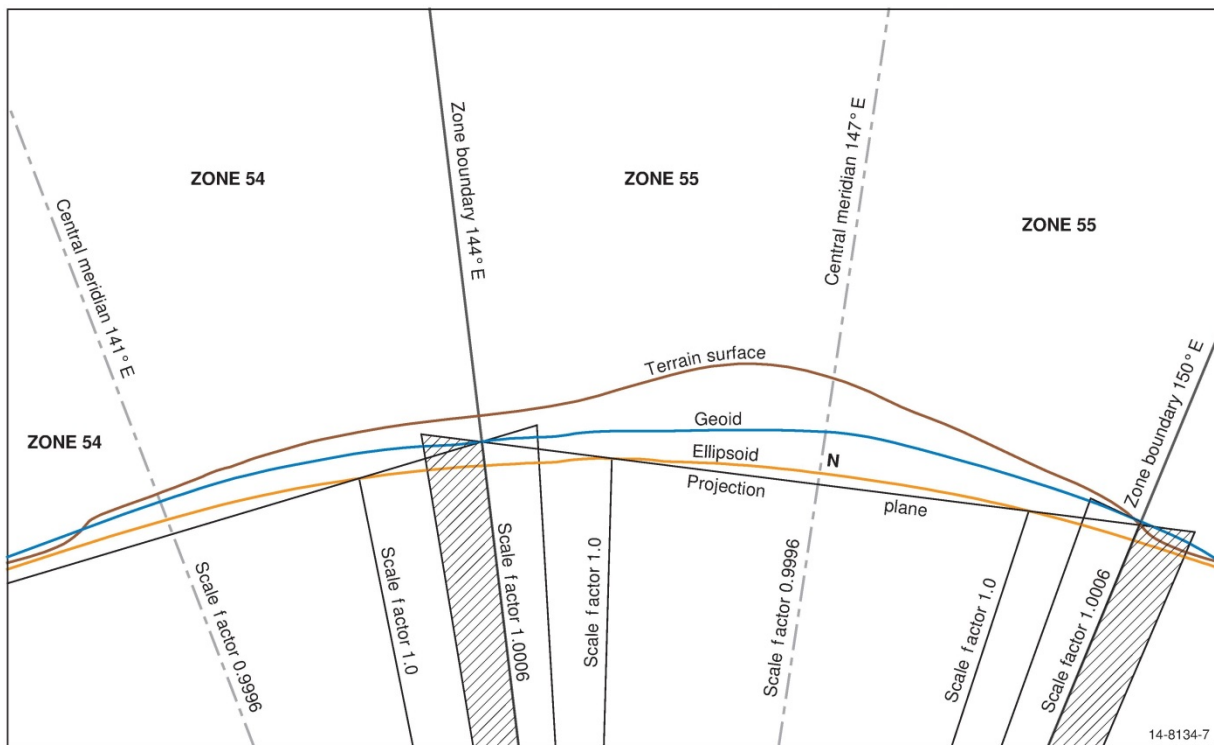
MGA cross section
